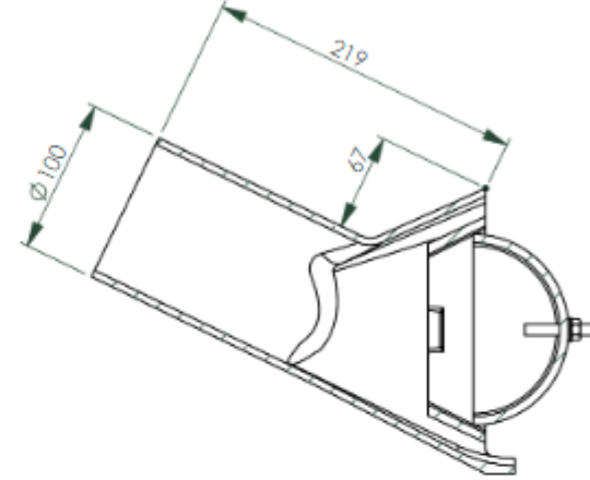
A-A (1 : 5)
