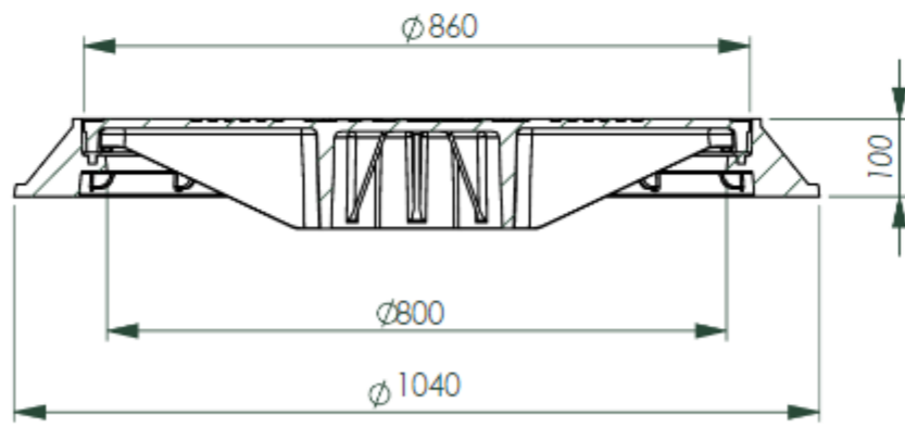
B-B (1 : 12)
