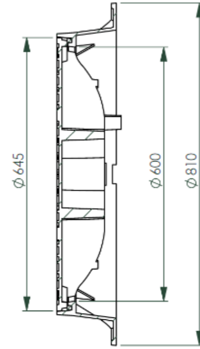
B-B
