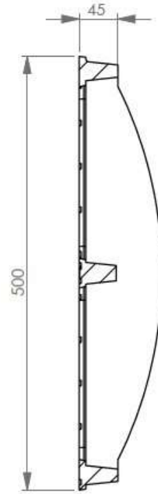
B-B (1 : 6)
