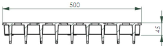
B-B (1 : 7)
