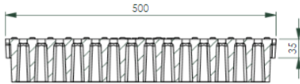
A-A (1 : 6)
