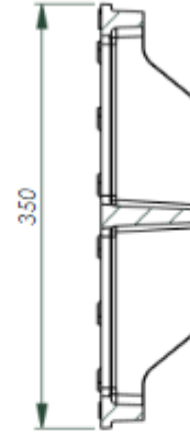
B-B (1 : 6)
