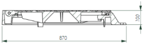
B-B (1 : 10)
