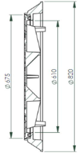
A-A (1 : 10)
