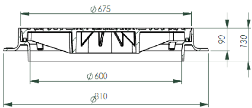
A-A (1 : 10)
