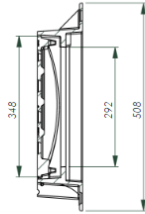
A-A (1 : 8)
