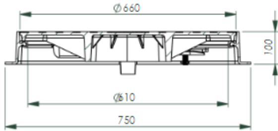
B-B (1 : 10)
